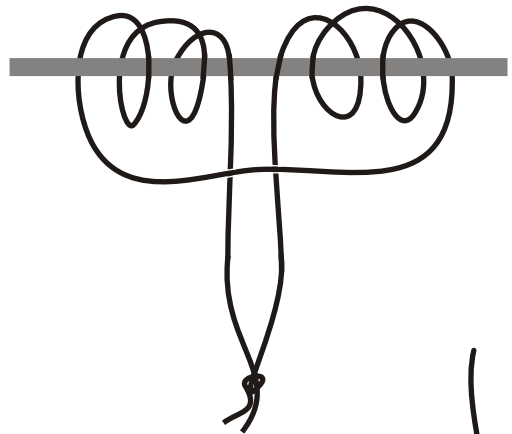
PRUSSIK KNOT
